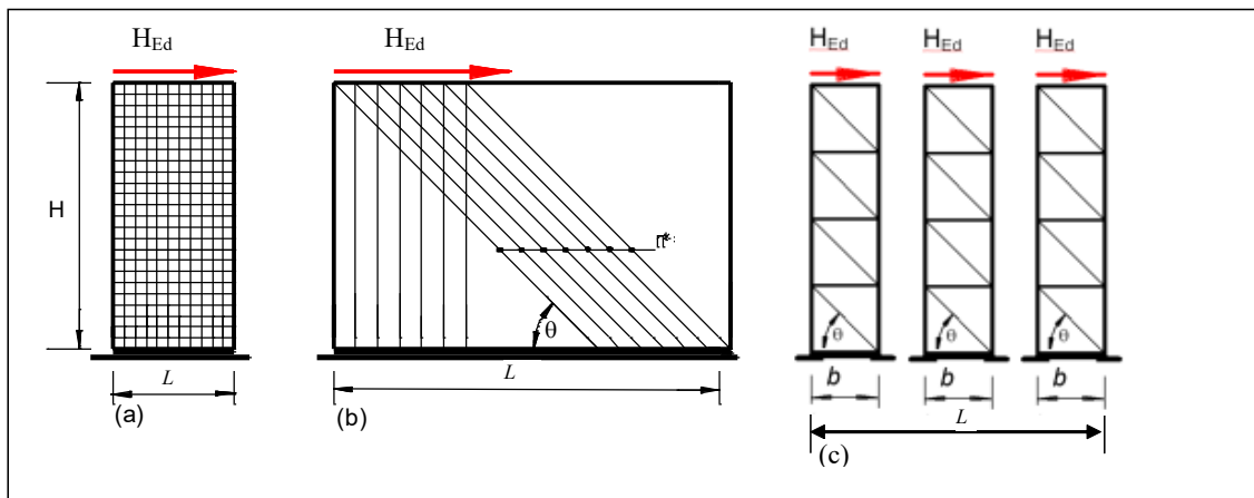
a) Rahmenmodell
